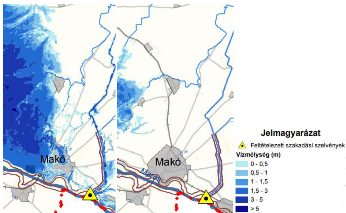
1-84. ábra: A település környezetének elöntési térképe 1%-os és 3,3%-os valószínűségű árvizek esetében
