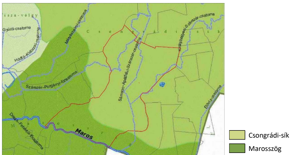
1-37. ábra: Makó elhelyezkedése a földrajzi tájbeosztás szerint
