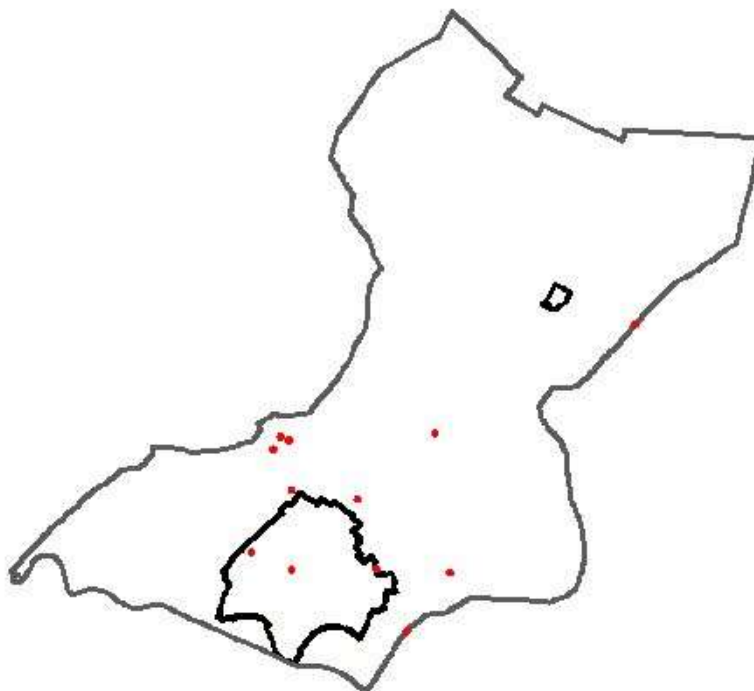
1-47. ábra: Ex lege védett kunhalmok
