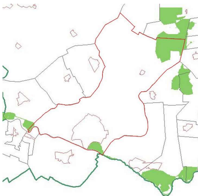
1-46. ábra: A Körös-Maros Nemzeti Park védett területei Makón
