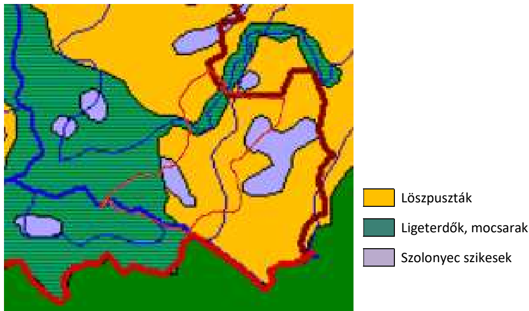
1-41. ábra: Természetes növénytakaró Makó térségében
