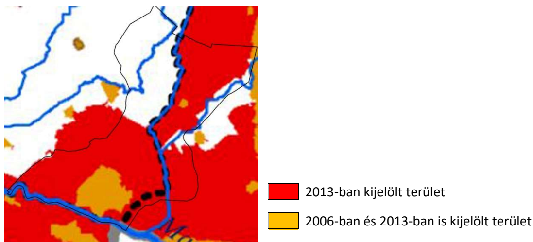
1-66. ábra: Nitrátérzékeny területek elhelyezkedése Makón
